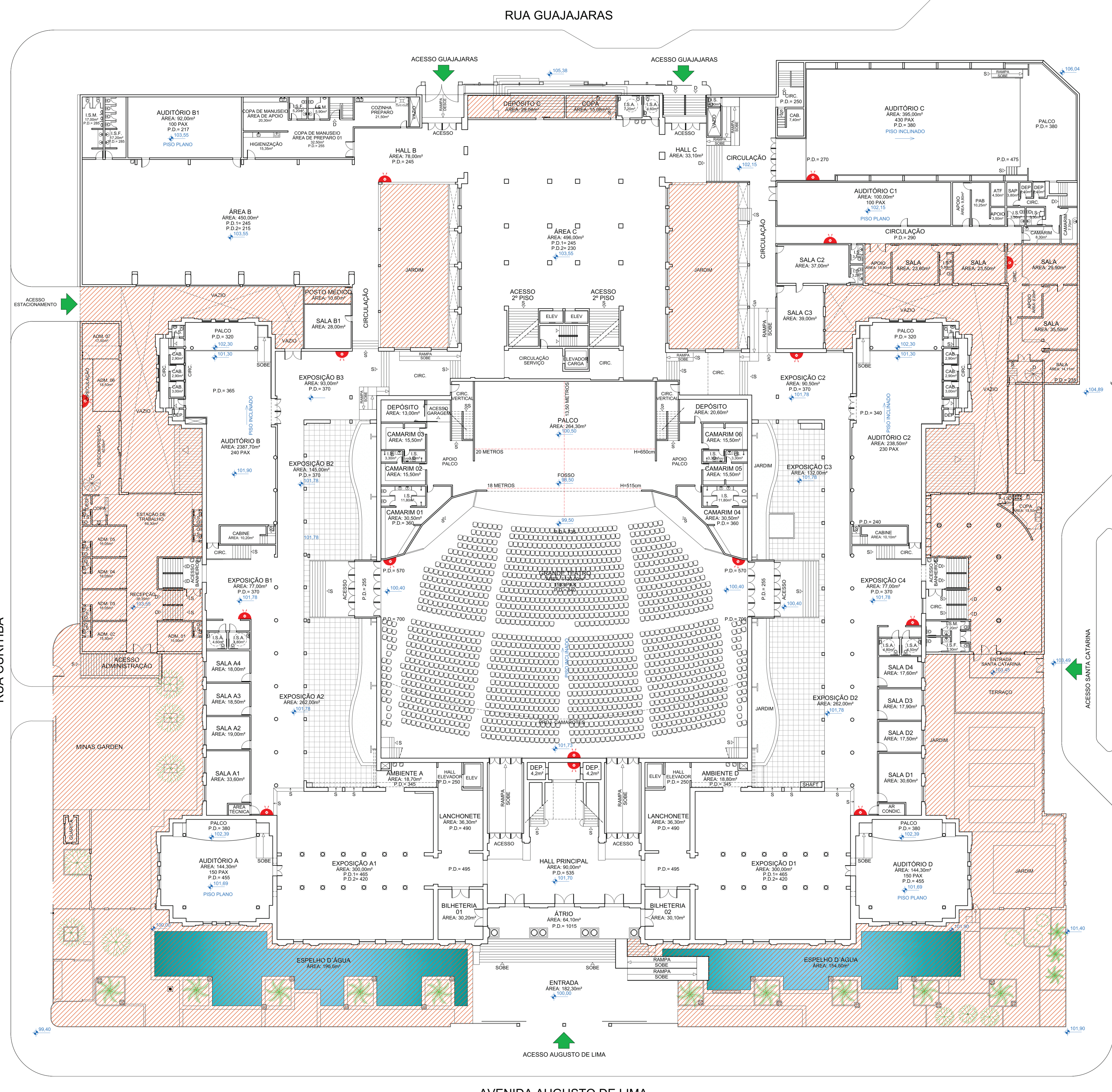
PLANTA 1º PAVIMENTO ESCALA 1/200
